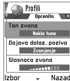
Slika 2 Postavke profila
