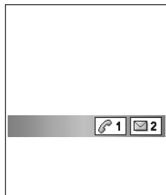
Slika 2 Čuvar zaslona.
