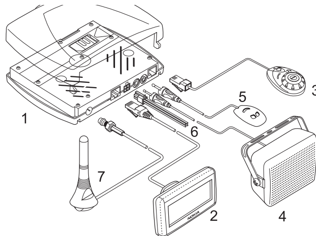
Комплект телефон за автомобил Nokia 610
