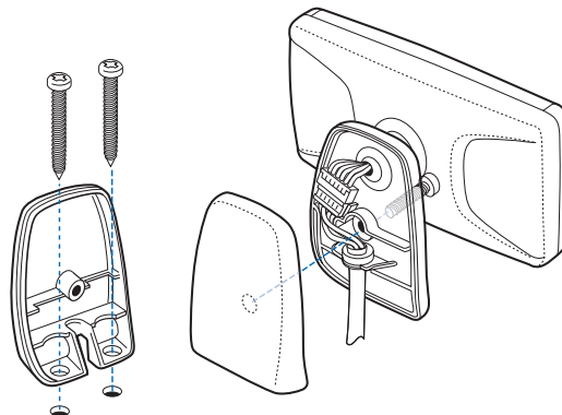
Как да монтирате дисплея
