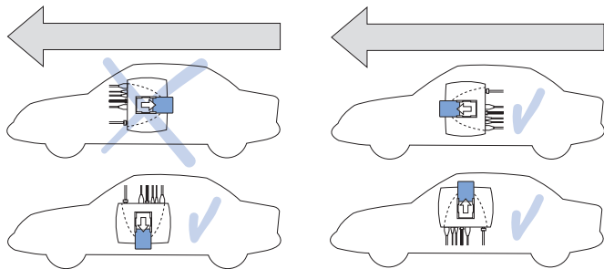
Как да монтирате радиоустройството в колата
