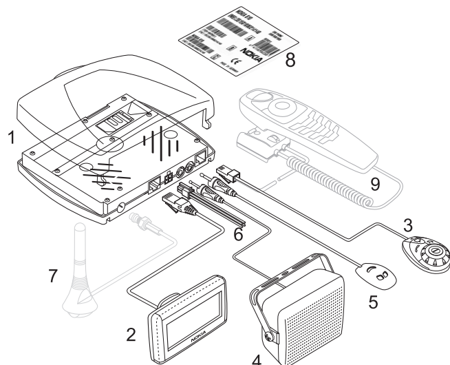
Εξοπλισμός του car kit Nokia 616
