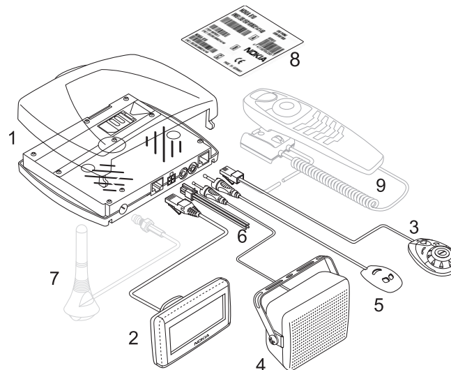
Εξοπλισμός και καλωδιακές συνδέσεις του car kit Nokia 616
