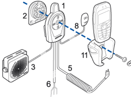
Pasif telefon tutucusuyla kullanılan araç kiti
