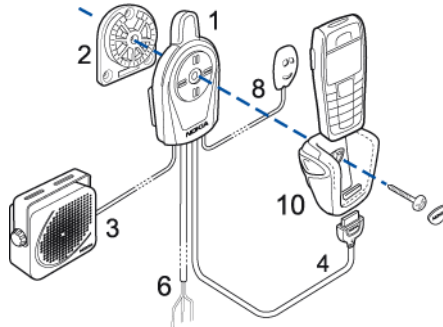
Aktif telefon tutucusuyla kullanılan araç kiti
