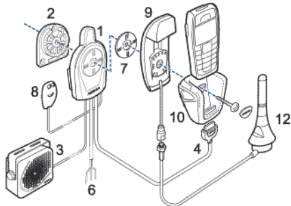
Ayrı anten bağlantı birimi ve harici anten kullanılan araç kiti
